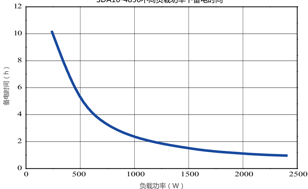
SDA10-4850不同负载功率下备电时间
