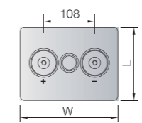
GFMJ-200~GFMJ-600
